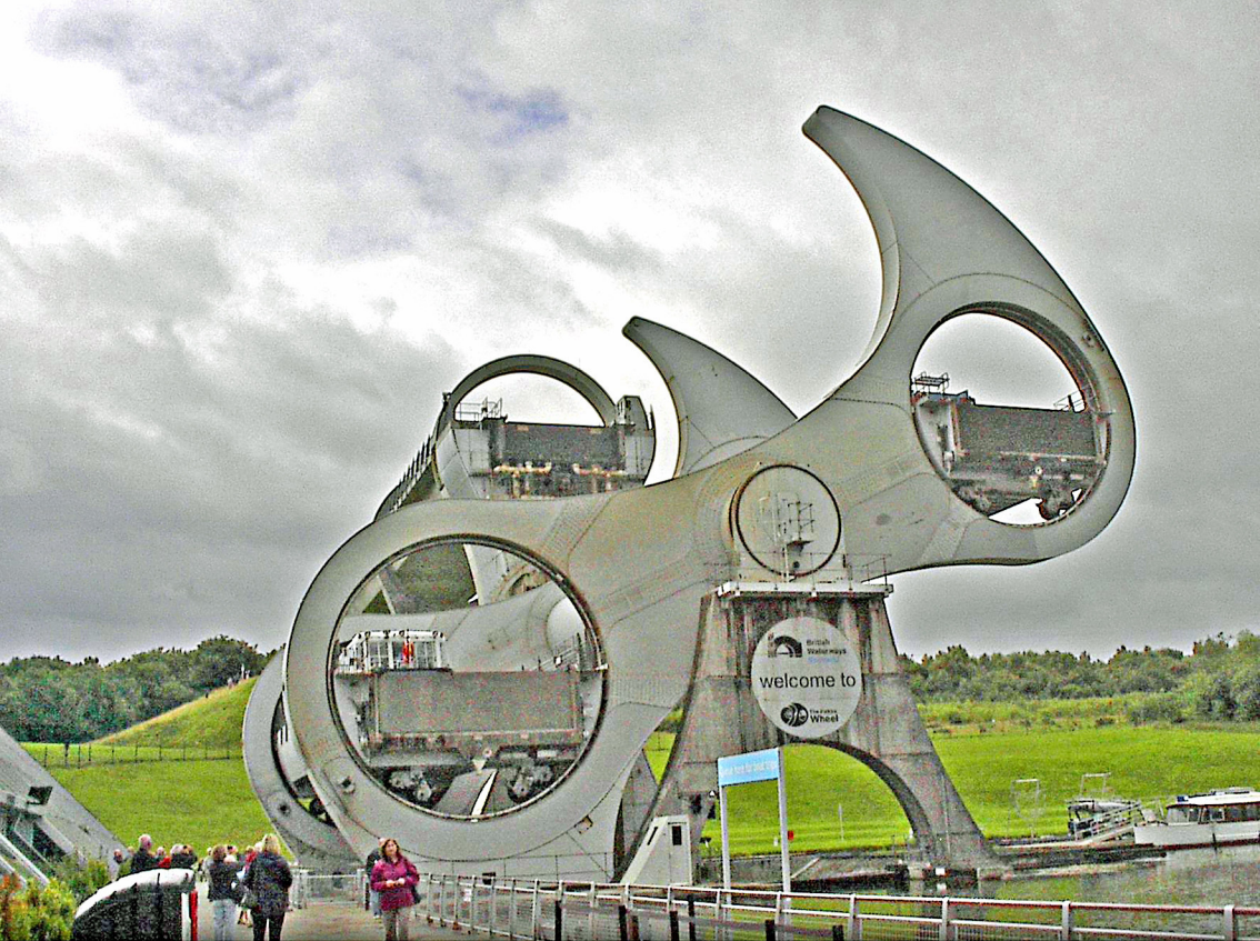
Falkirk-Wheel - die beiden Wannen sind weiter gedreht
